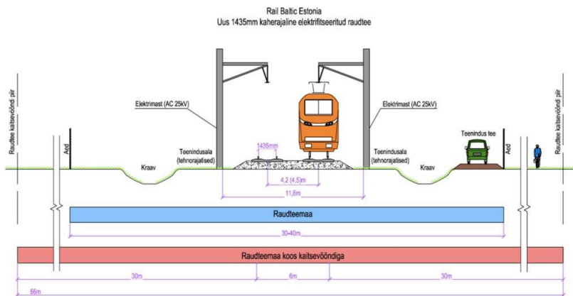
Joonis-foto: Kavandatud kaheajalise elektrifitseeritud raudtee kaitsevööndi lõige trassikoridoris. 33
